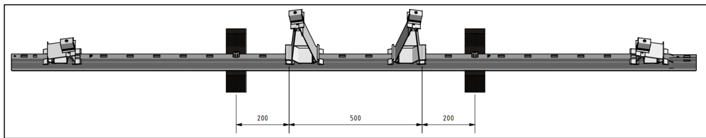
Vue de côté 2500mm pitch
