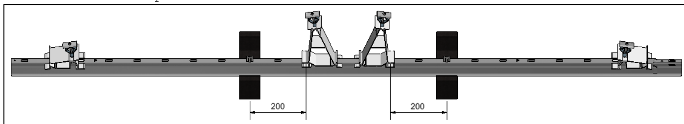
Vue de côté: 2300mm pitch
