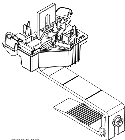
729503 ValkAce+ - Slimline dakhaak - verstelbaar 35-59mm
