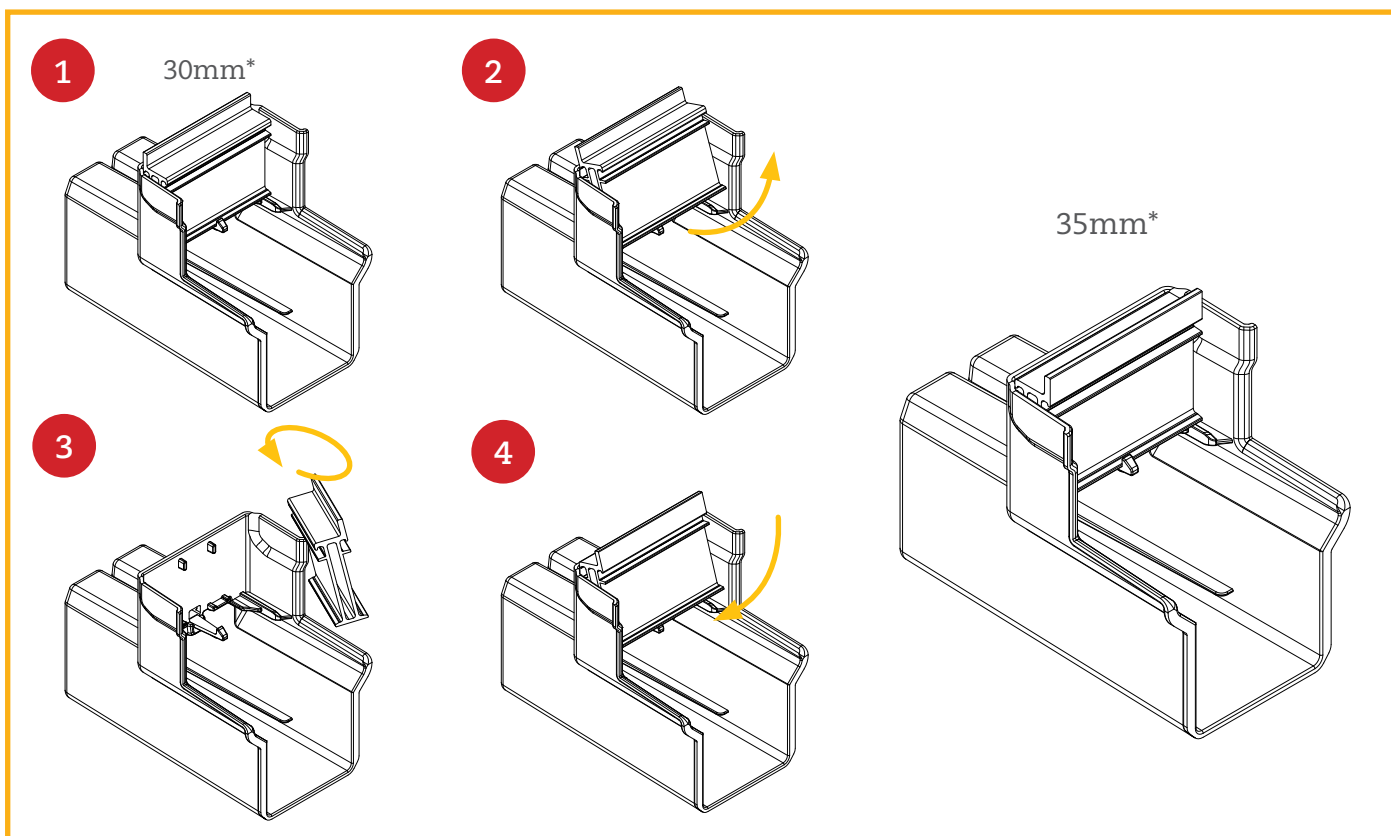
770230 (30mm) ValkGrip
