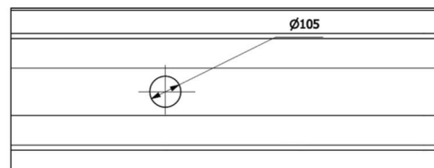
ValkTop - Dakgoot Double - Eindstuk met gat
